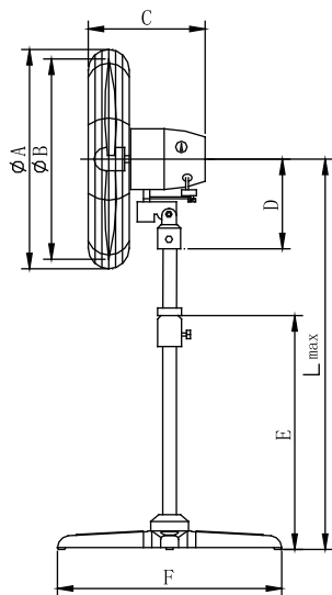
Ventilador Pedestal
